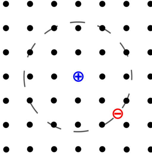
Şekil 1. Egzitonlar, elektron ve hole'ların oluşturduğu, Hidrojen atomu benzeri kararlı yapılarıdır
