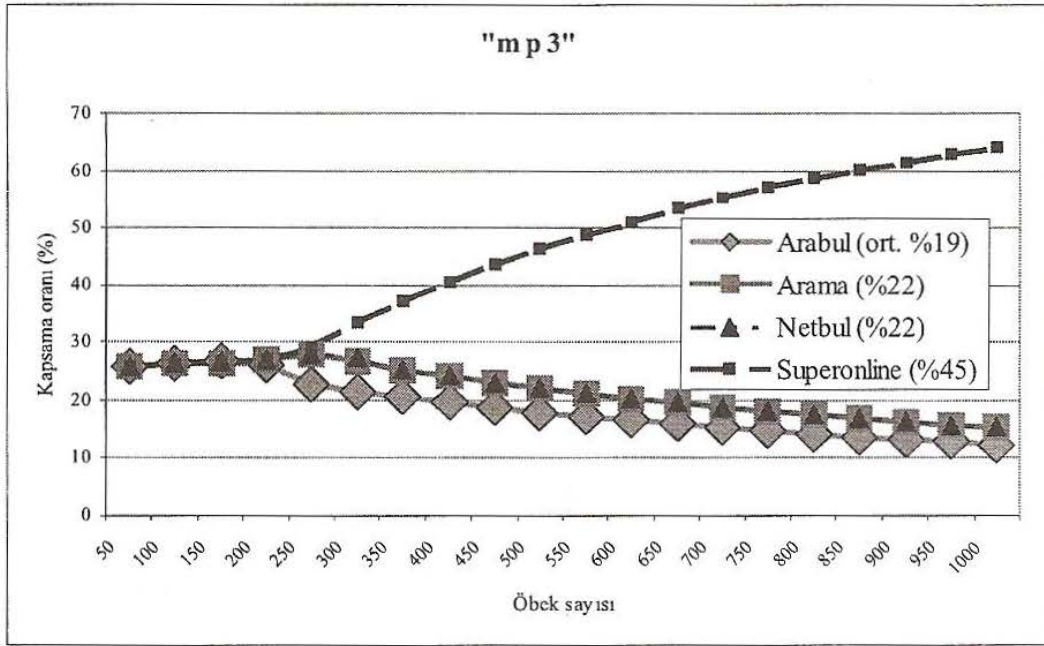
Şekil 11. Arama motorlarının "mp3" için öbekteki belge sayısına göre kapsama oranları
