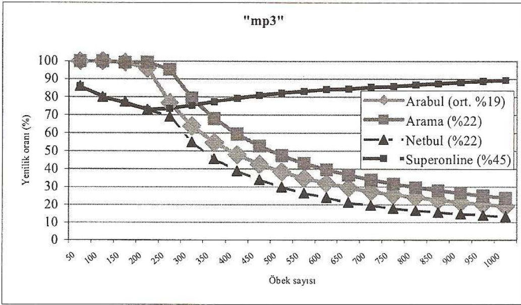
Şekil 16. Arama motorlarının "mp3" sorusu için yenilik oranları
