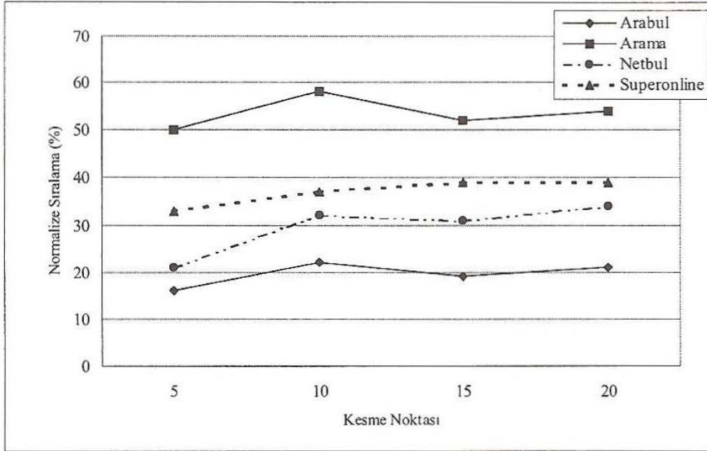
Şekil 9. Ortalama normalize sıralama değerleri
