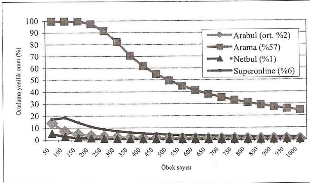
Şekil 19. Arama motorlarının tüm sorular için Türkiye adresli yeni belge bulma oranları
