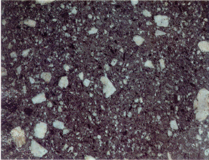
Porfiritik-afanitik doku
