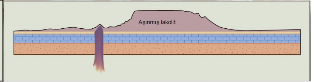
Aşınmış lacolit
