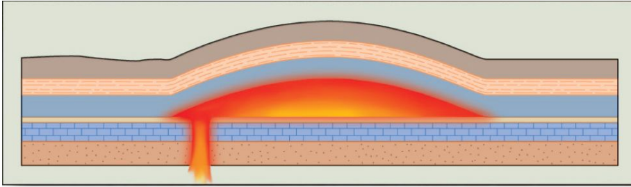
Lacolit
