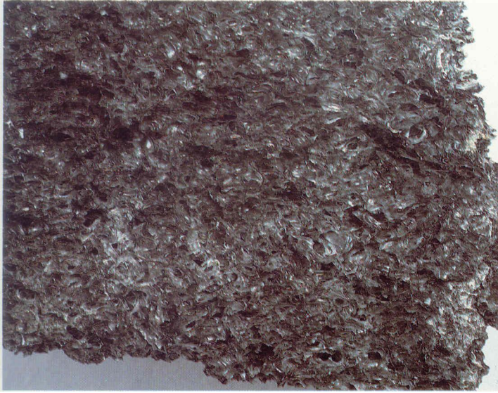
Camsı doku
