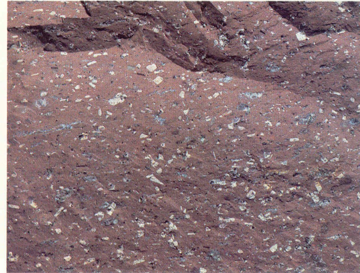
Porfiritik-afanitik doku
